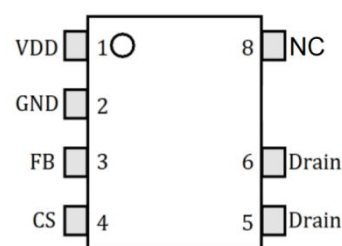
SOP-7俯视图
